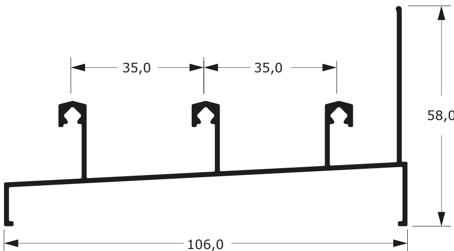
DSU-219 0,999 Kg/m
