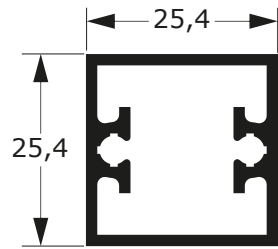
D-080 0,525 Kg/m
