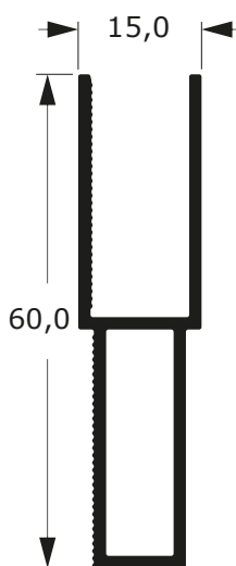
78-2250C 0,591 Kg/m
