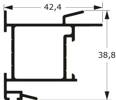
DSU-042 0,589 Kg/m
