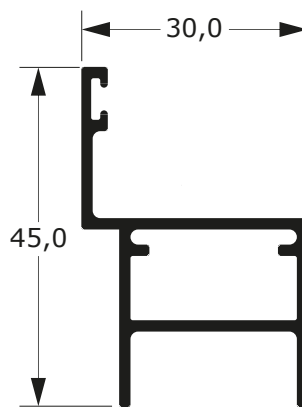
P-155 0,528 Kg/m
