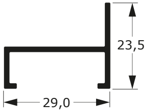
Y-120 0,263 Kg/m (25-557)
