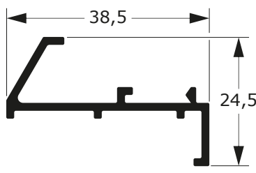
Z-063 0,325 Kg/m
