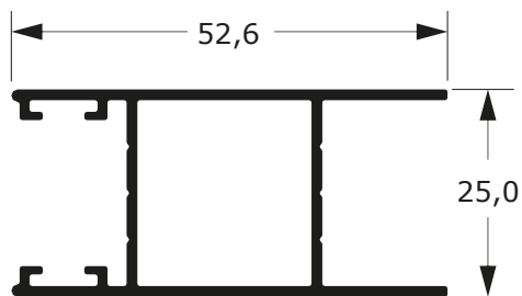
DSU-068 0,574 Kg/m
