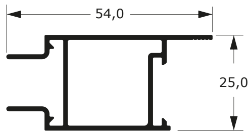
DSU-192 0,554 Kg/m
