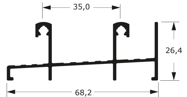
MG25-578 0,707 Kg/m
