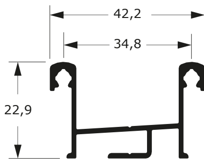
MG25-272 0,434 Kg/m
