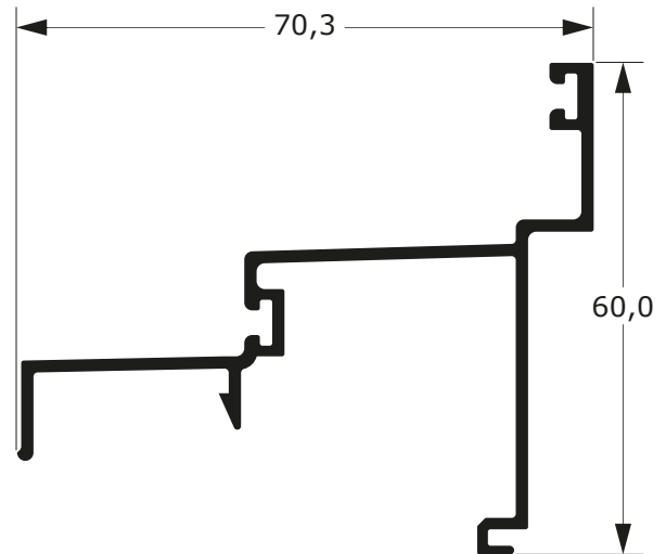
FC-222 0,757 Kg/m
