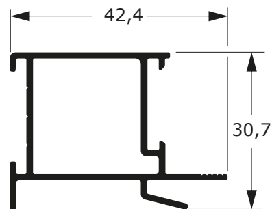
DSU-040 0,482 Kg/m
