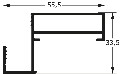
FC-293 0,683 Kg/m
