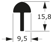
G-021 0,172 Kg/m
