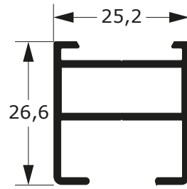
SU-091 0,401 Kg/m
