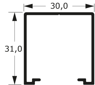
31-137C 0,339 Kg/m
