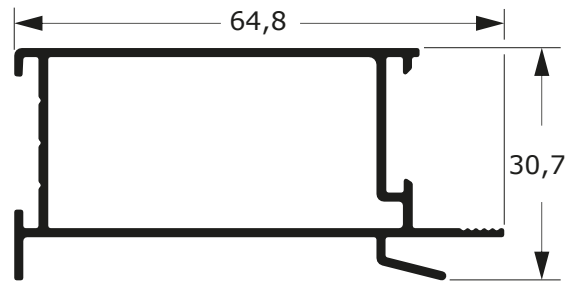
DSU-243 0,636 Kg/m
