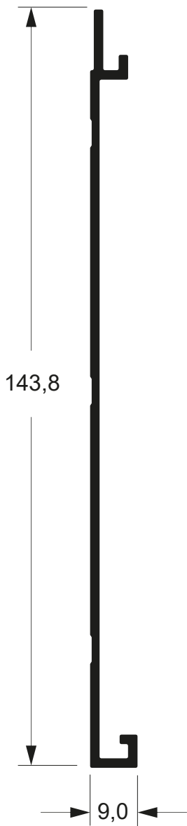
MG25-380 0,794 Kg/m
