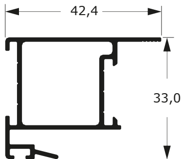
DSU-041 0,532 Kg/m
