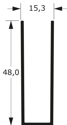
PU-200 0,409 Kg/m
