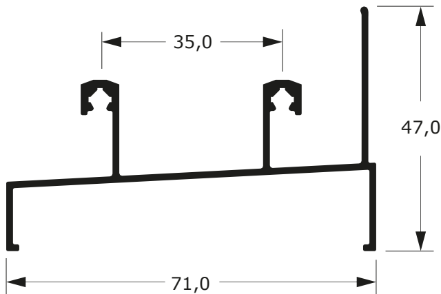
DSU-002 0,710 Kg/m
