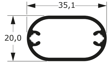
78-366 0,388 Kg/m
