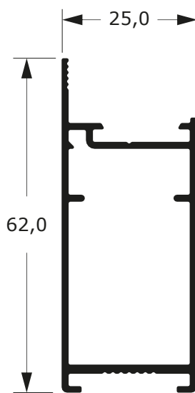
DSU-111 0,634 Kg/m
