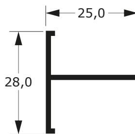
T-095 0,204 Kg/m
