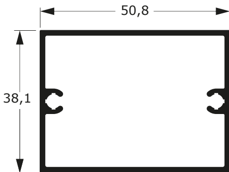
D-103 0,786 Kg/m
