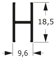
39-2072C 0,145 Kg/m
