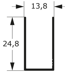
PU-104L 0,133 Kg/m
