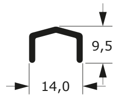
MG32-086 0,114 Kg/m
