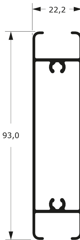
MG25-790 0,971 Kg/m
