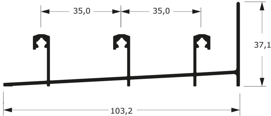
DSU-230 0,976 Kg/m
