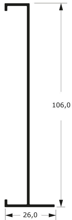
SU-012 0,539 Kg/m
