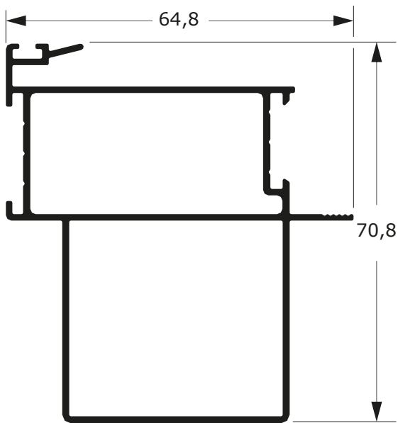
DSU-290 1,078 Kg/m
