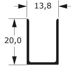
BX-102 0,126 Kg/m
