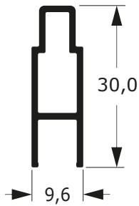
78-2302C 0,242 Kg/m
