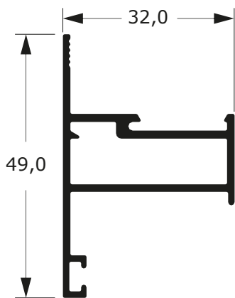
DLG-085 0,533 Kg/m
