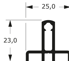
DSU-271 0,347 Kg/m
