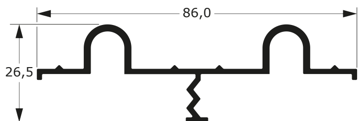
E-365 0,656 Kg/m
