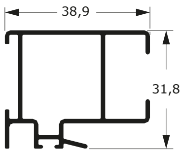
DSU-056 0,538 Kg/m
