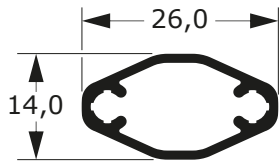
78-1021 0,248 Kg/m
