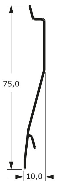
Z-201 Furada: Z-201F 0,263 Kg/m
