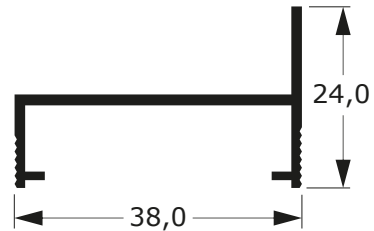
CM-060 0,223 Kg/m
