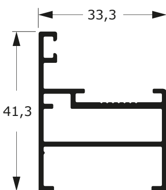
DSU-279 0,565 Kg/m
