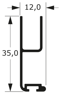
39-2398C 0,244 Kg/m
