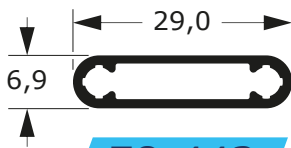
78-442 0,226 Kg/m
