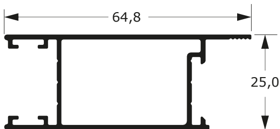
DSU-245 0,636 Kg/m
