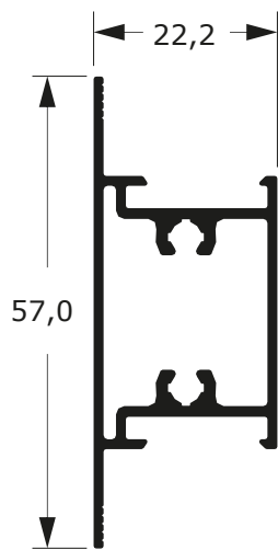
DSU-227 0,574 Kg/m
