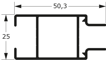
SU-190 0,543 Kg/m
