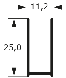
BX-114 0,159 Kg/m
