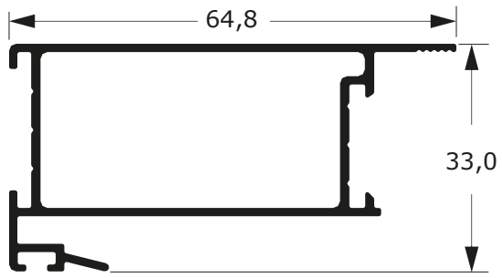
DSU-242 0,674 Kg/m
