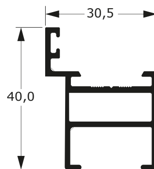
P-412 0,453 Kg/m
