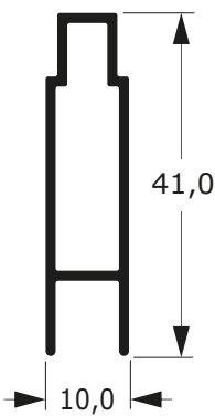
78-2465C 0,316 Kg/m
