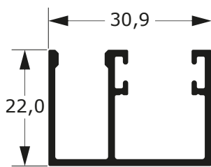
EX-306L 0,388 Kg/m
