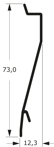
VZ-051 Furada: VZ-051F 0,265 Kg/m
