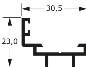
L-715 0,293 Kg/m
