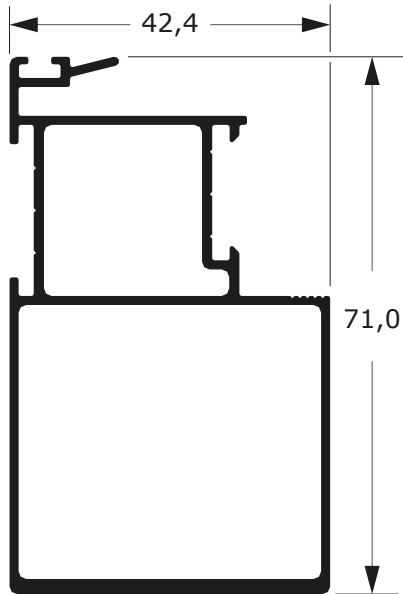
DSU-049 0,997 Kg/m
