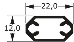
D-070 0,256 Kg/m
