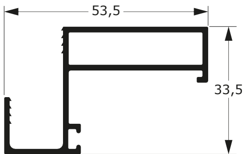
78-043 0,631 Kg/m
