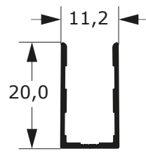
BX-101 0,114 Kg/m
