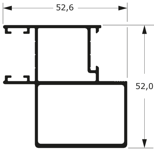
DSU-044 0,957 Kg/m
