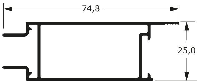
DSU-244 0,699 Kg/m
