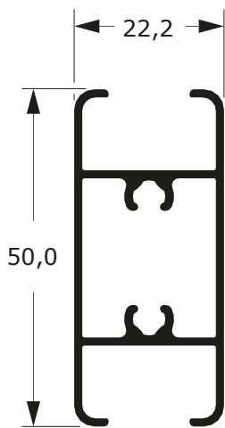
DSU-188 0,586 Kg/m
