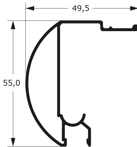
BX-117 0,558 Kg/m
