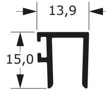
EX-1091 0,176 Kg/m
