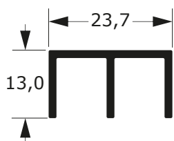
E-168 0,236 Kg/m
