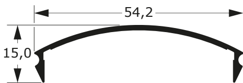
CG-074 0,267 Kg/m
