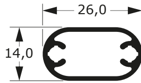
78-1017 0,286 Kg/m
