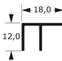
F-049 0,128 Kg/m
