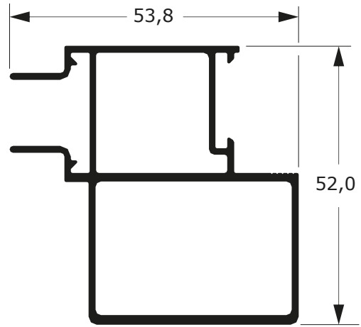
DSU-043 0,947 Kg/m
