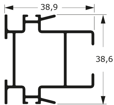
DSU-057 0,632 Kg/m
