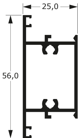
P-319 0,657 Kg/m
