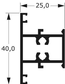
P-153 0,598 Kg/m
