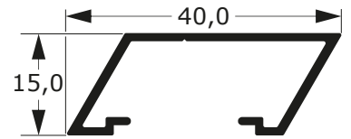
39-2370C 0,275 Kg/m
