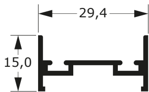
I-105 0,259 Kg/m
