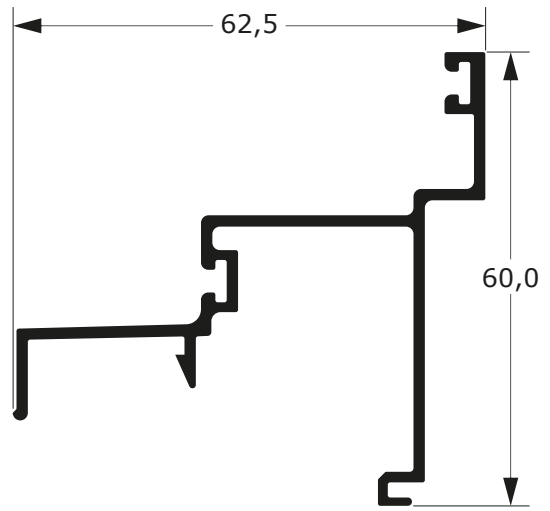
39-487 0,738 Kg/m
