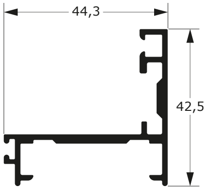
FC-225 0,639 Kg/m
