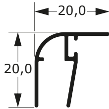
BX-105 0,166 Kg/m
