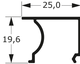
39-2073C 0,219 Kg/m
