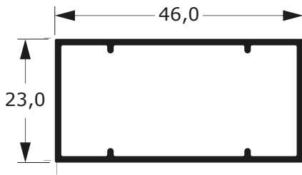
78-952 0,451 Kg/m
