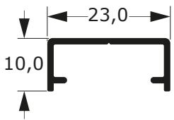
31-128C 0,147 Kg/m
