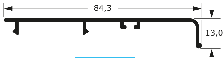
FC-229 0,464 Kg/m
