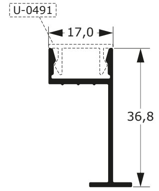
U-0491 0,093 Kg/m
