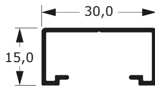
31-138C 0,235 Kg/m
